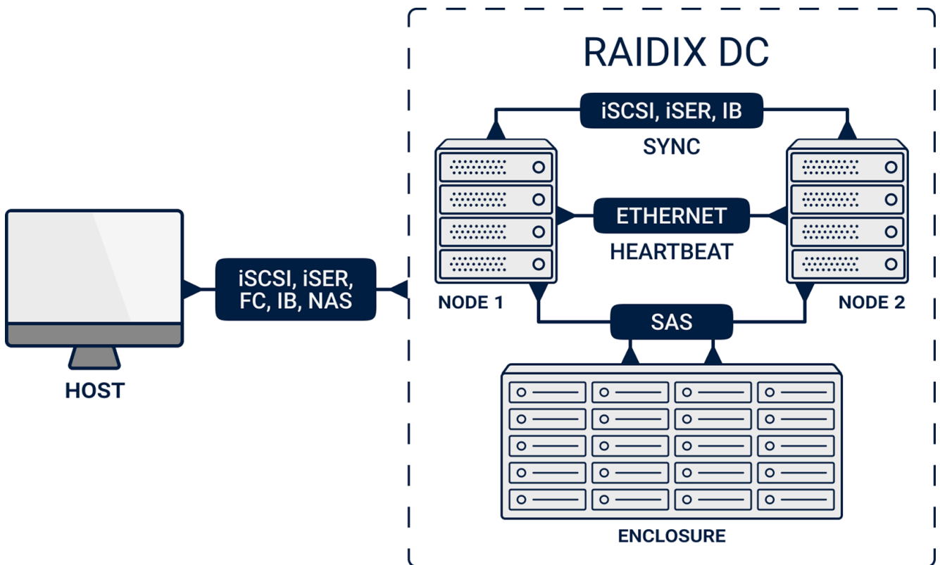
Рис. 2. Схема двухконтроллерного режима работы системы RAIDIX 5.2.5
