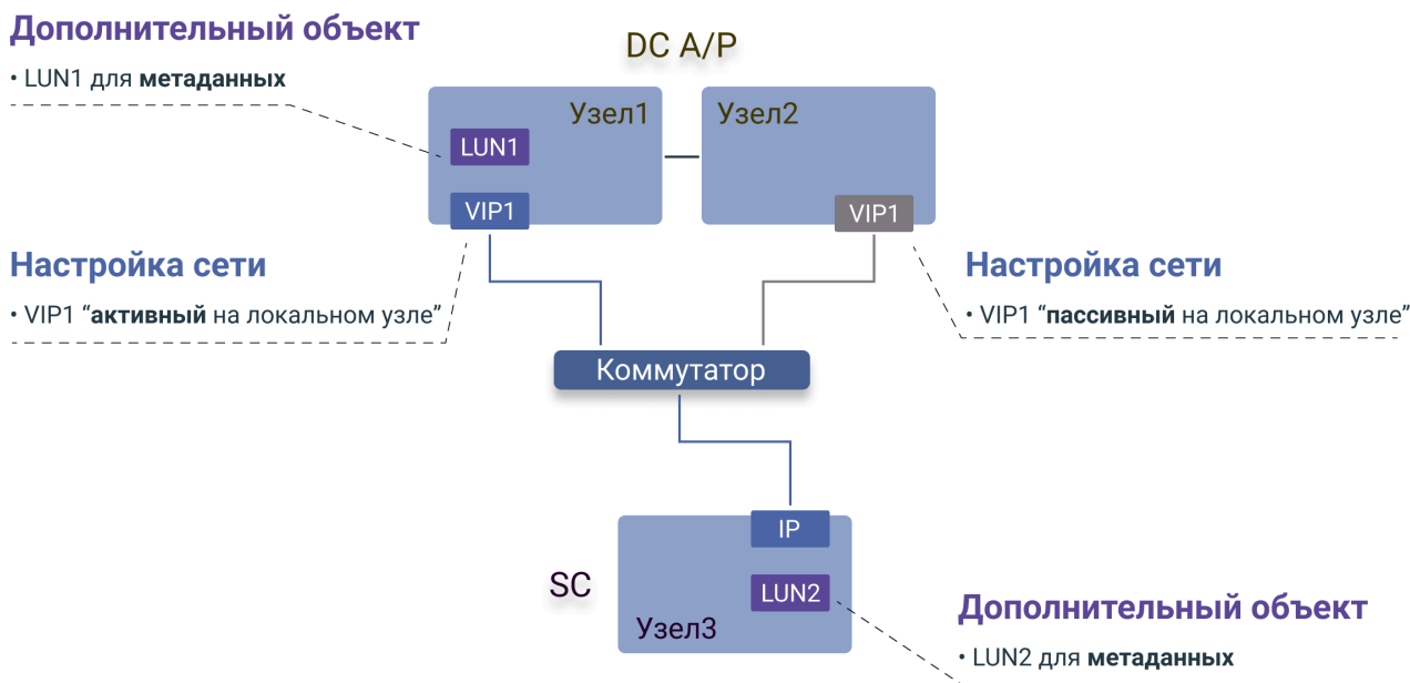
Рис. 67. Схема СХД для репликации с DC Active/Passive на SC
