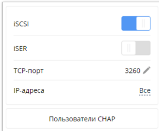
Рис. 110. Переключатель «iSCSI»
