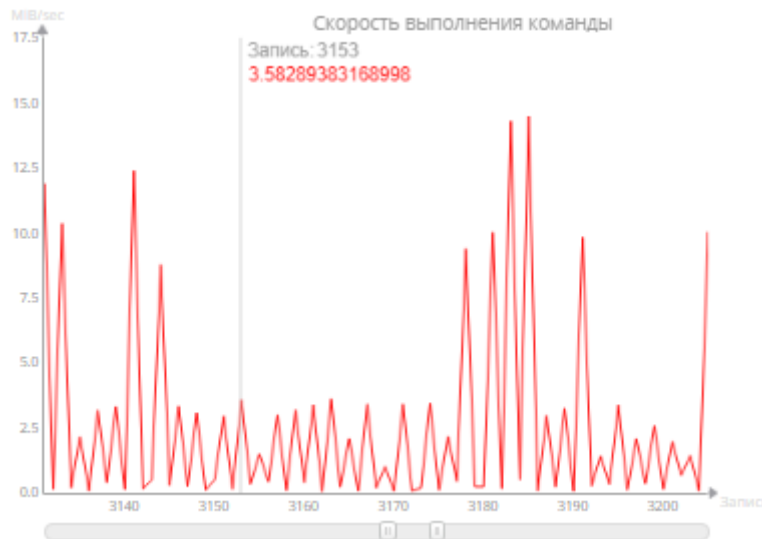
Рис. 170. Пример графика «Скорость выполнения команды»
