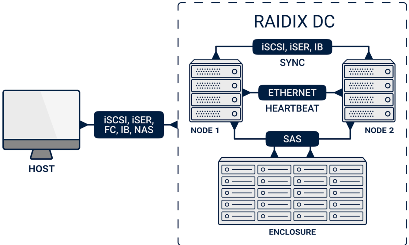
Рис. 2. ПО RAIDIX 5.2.5: Двухконтроллерный режим работы
