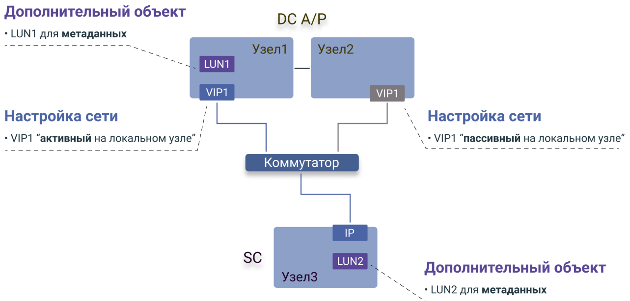
Рис. 66. Схема СХД для репликации с DC Active/Passive на SC
