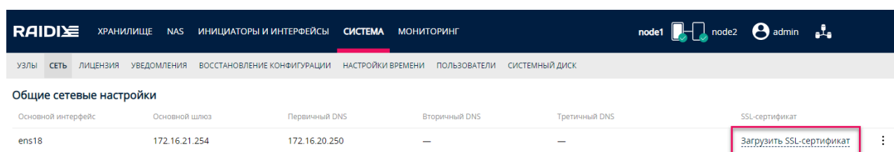
Рис. 127. Загрузка SSL-сертификата
