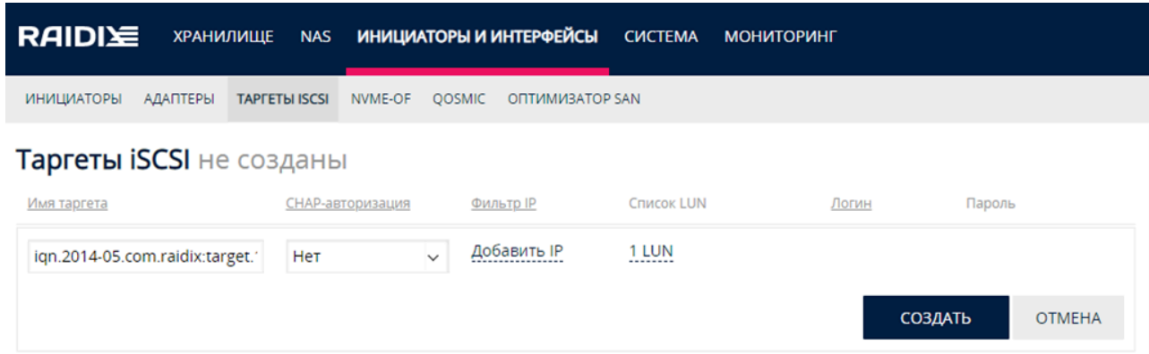
Рис. 95. Виджет создания iSCSI-таргета
