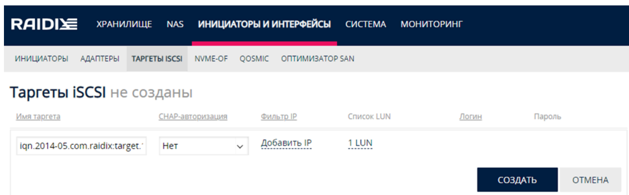
Рис. 16. Страница ТАРГЕТЫ ISCSI. Виджет создания таргета
