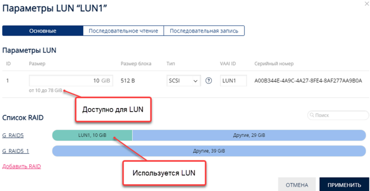
Рис. 50. Параметры LUN после добавления Generic RAID
