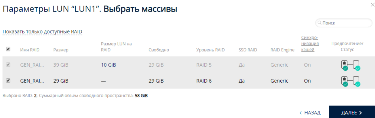
Рис. 49. Выбор RAID, которые будут добавлены к LUN
