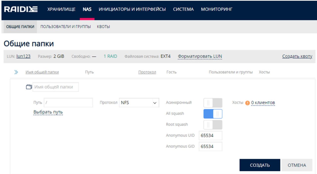
Рис. 78. Виджет создания общей папки с выбранным протоколом NFS
