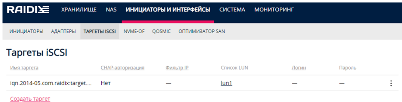
Рис. 17. Страница ТАРГЕТЫ iSCSI. Список таргетов
