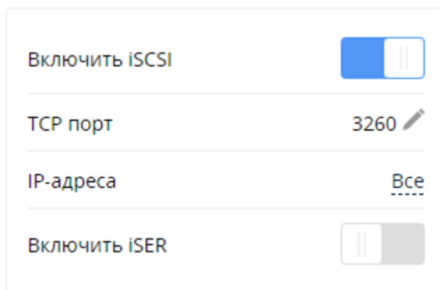
Рис. 15. Страница ТАРГЕТЫ ISCSI. Переключатель «Включить iSCSI»
